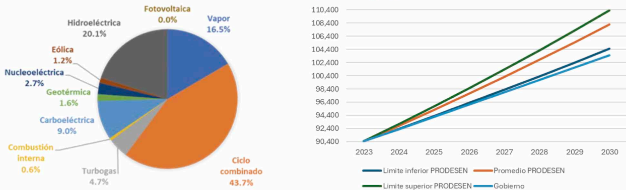
Izq. México. Contribución a la capacidad instalada por tipo de tecnología 2023 (porcentaje)/ Der. México. Capacidad instalada total por años proyectados.
